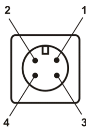
Рисунок 3.3 Разъем подключения преобразователя влажности
