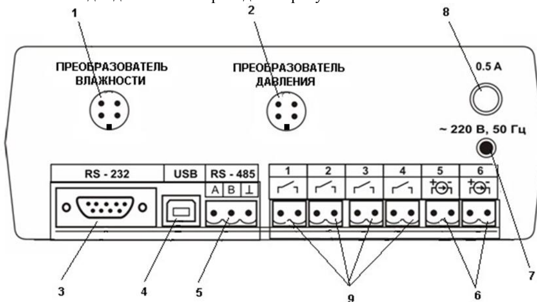
Рисунок 3.2 Задняя панель прибора
