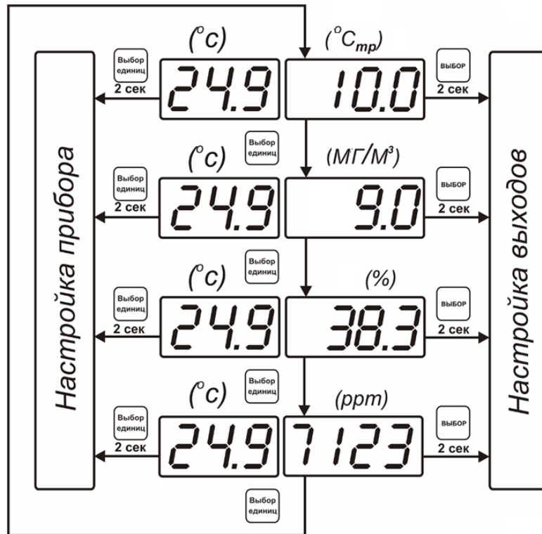
Рисунок 6.1 Режим РАБОТА
