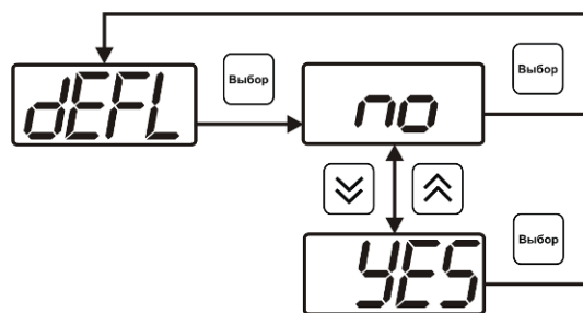
Рисунок 6.15 Возврат к заводским установкам
