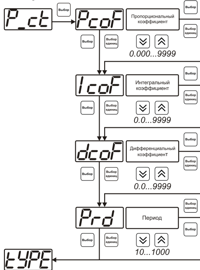
Рисунок 6.24 Настройка коэффициентов ПИД-регулятора (реле)
